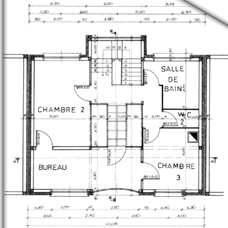
PLAN R+2
